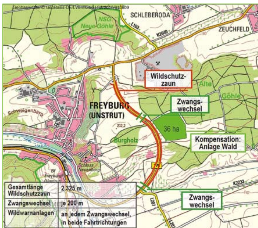
Wildwarnanlage an der Ortsumgebung Freyburg.
