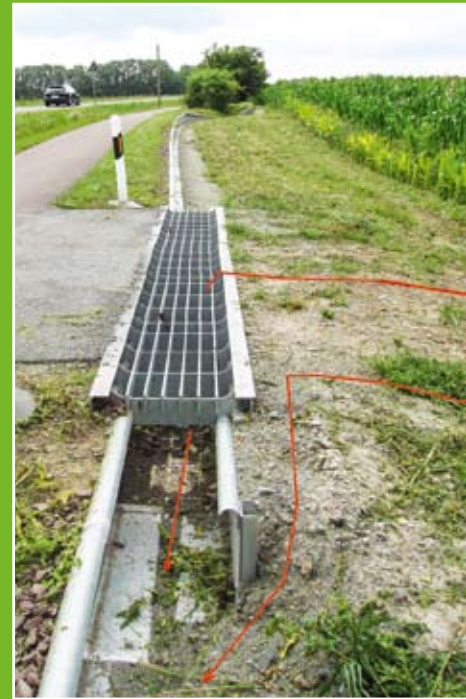
An Einmündungen von Wegen auf die Straße werden sogenannte Stopprinnen eingebaut. Die Gitter stellen einen unattraktiven Untergrund für Amphibien dar. Wegen die Tiere dennoch eine Überquerung, fallen sie durch die Gitter und landen wieder an der Leiteinrichtung. (Anlage B 188 bei Solpke)
