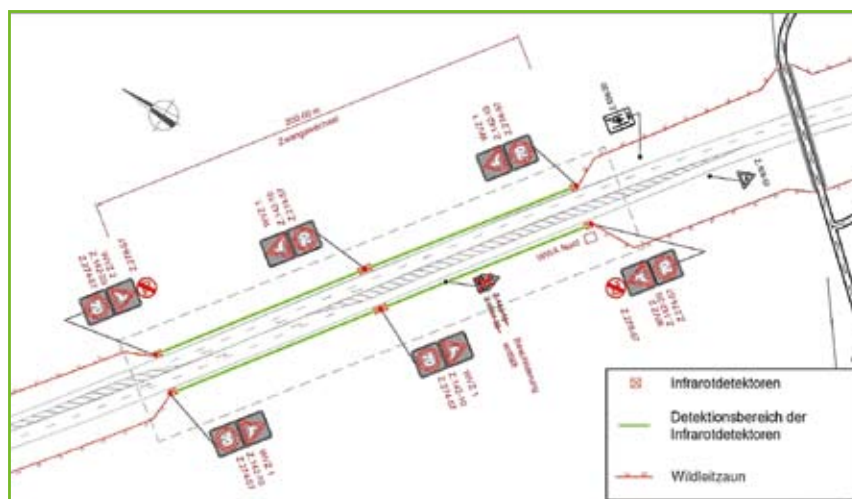
B 176 OU Freyburg: Auszug aus dem Bauplan (Maßnahme Nr. 15): Nördlicher Zwangswechsel mit Wildschutzzaun, Zwangswechselbereich und den Standorten der Signaltafeln.
